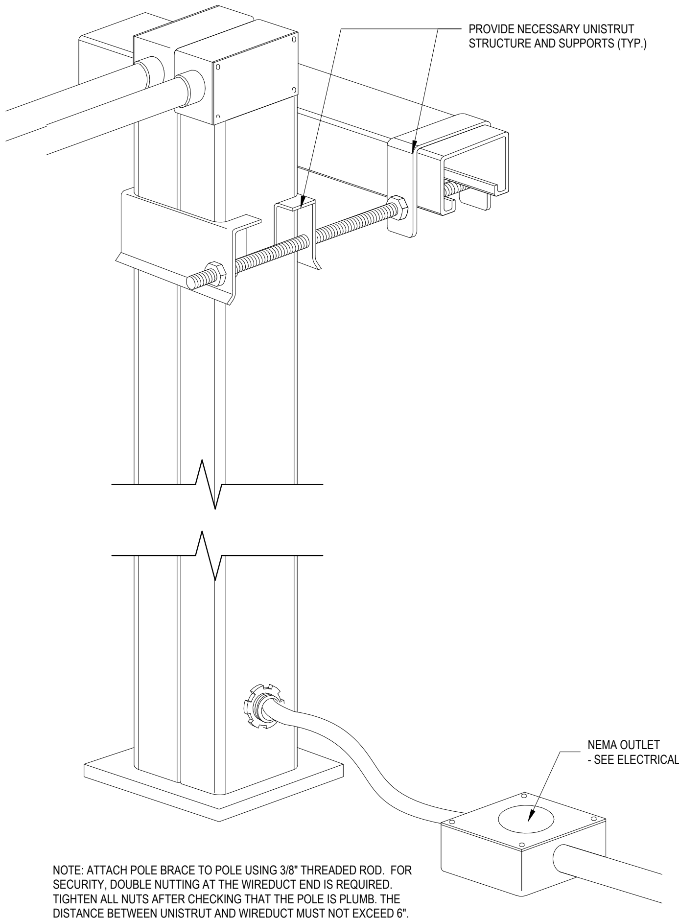
D5 POWER POLE N.T.S.
