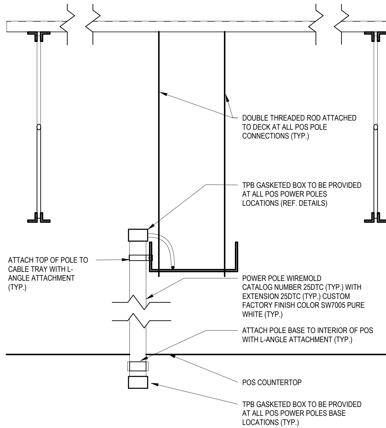
E5 POS POWER POLE N.T.S.
