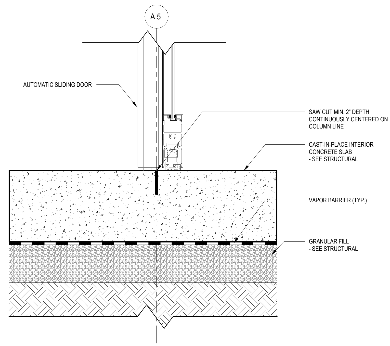
E4 SILL @ VESTIBULE DOOR 3" = 1'-0"
