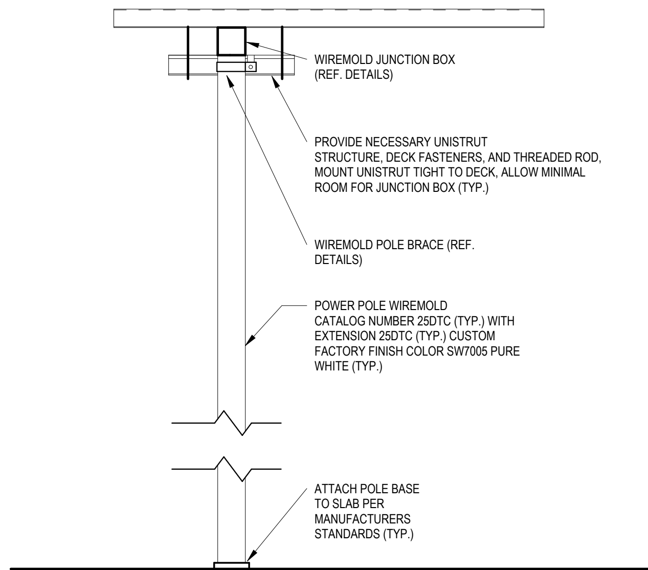
E3 POWER POLE N.T.S.
