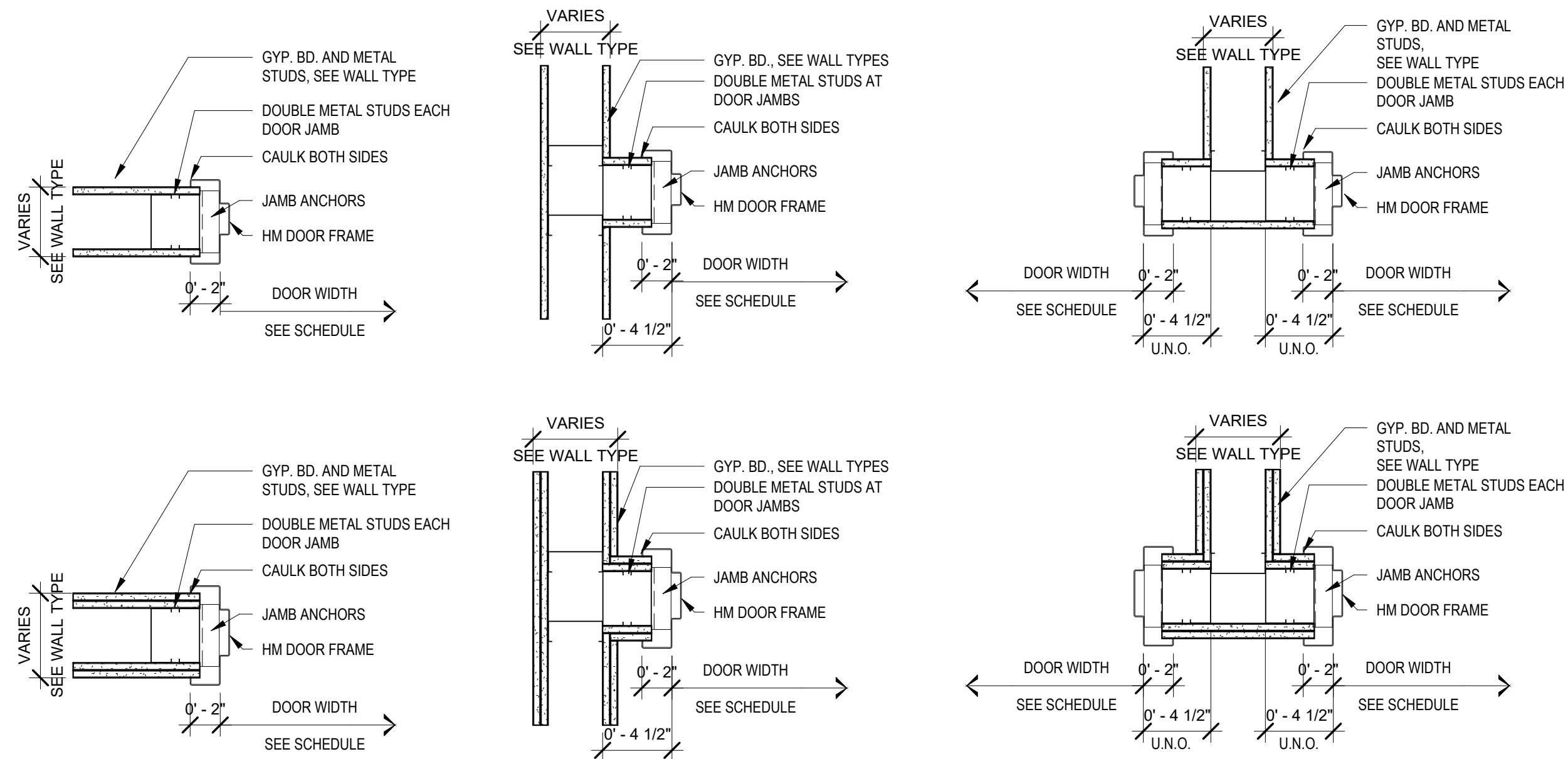
C2 TYP. HM DOOR JAMB 1 1/2" = 1'-0"
